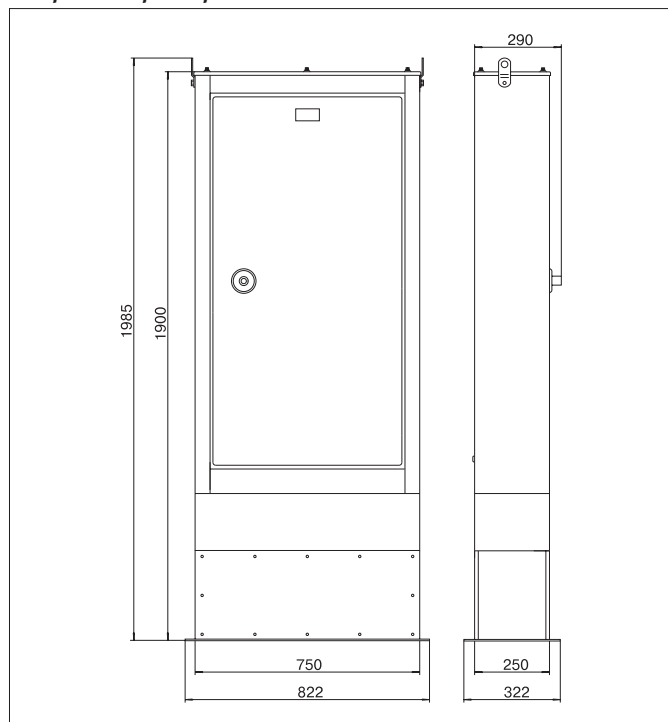
Габаритные размеры ШУО
