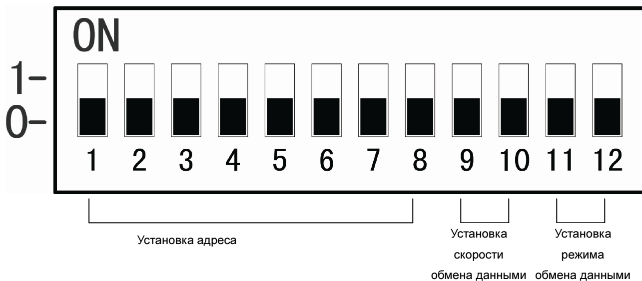
Рисунок 5.1. DIP-переключатель
