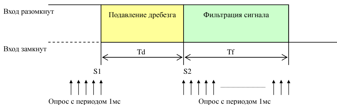
Рисунок 5.2. Подавление дребезга и фильтрация сигнала на входе
